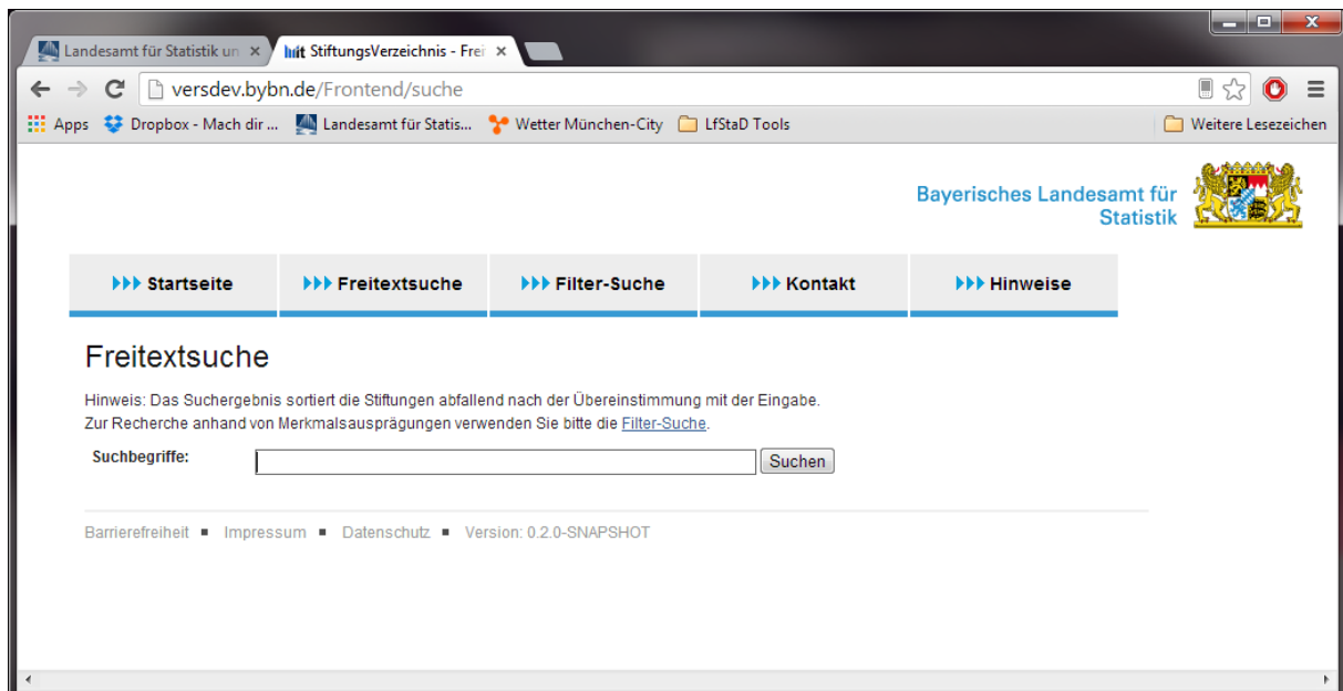
Abbildung 1: Dialog: Freitextsuche
