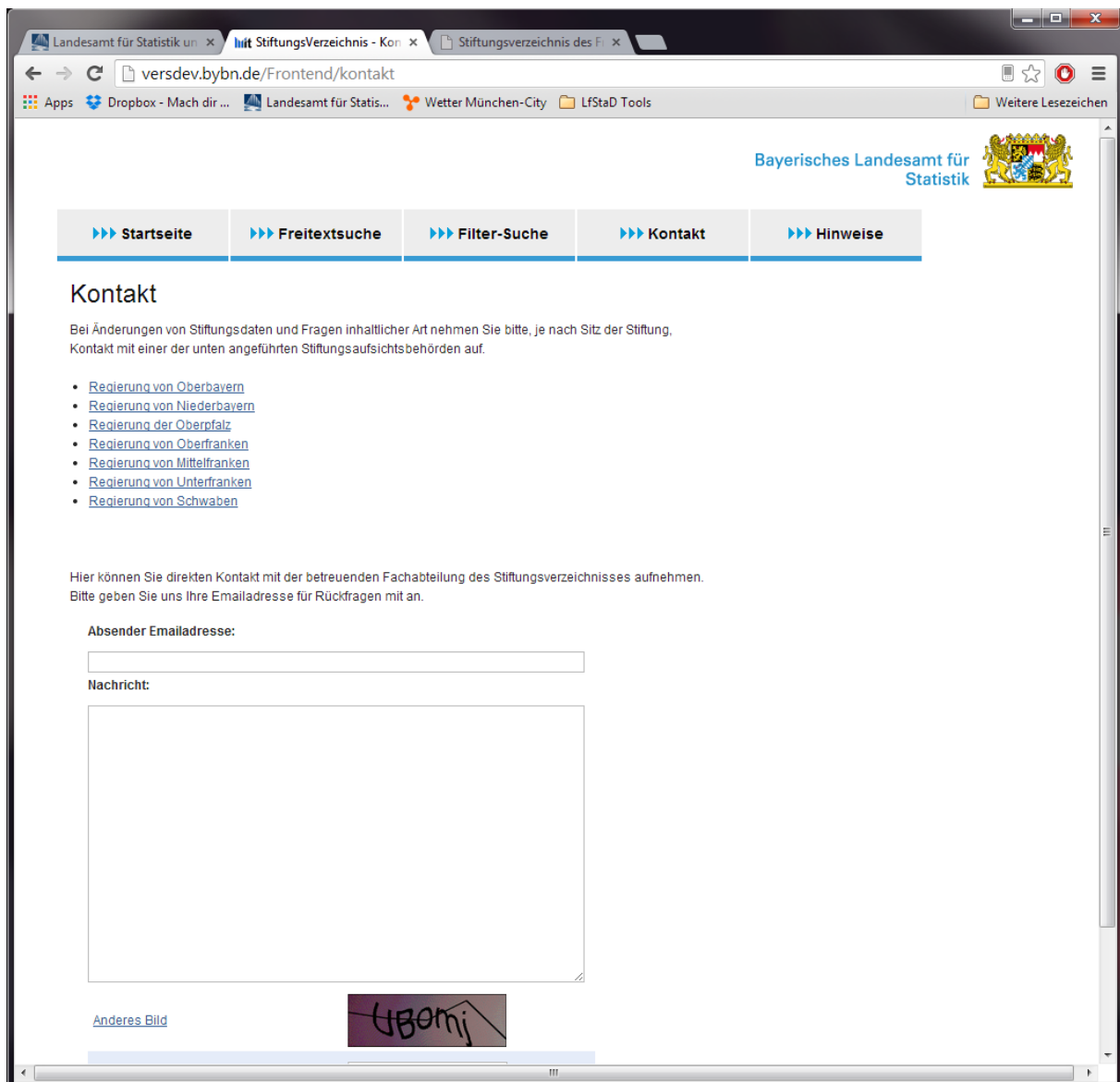
Abbildung 4: Dialog "Kontakt"
