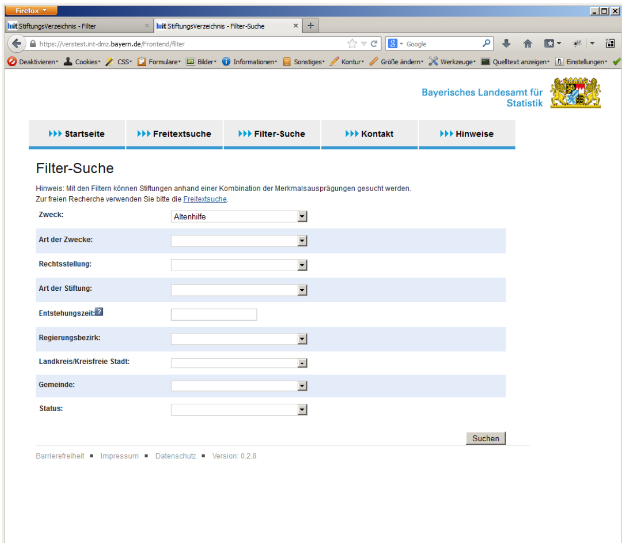
Abbildung 2: Dialog "Filter-Suche"
